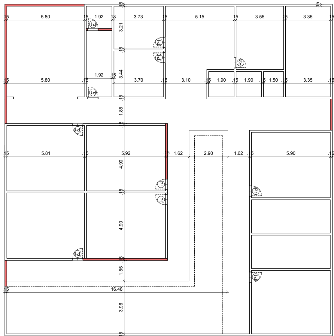
PLANTA ATUAL
