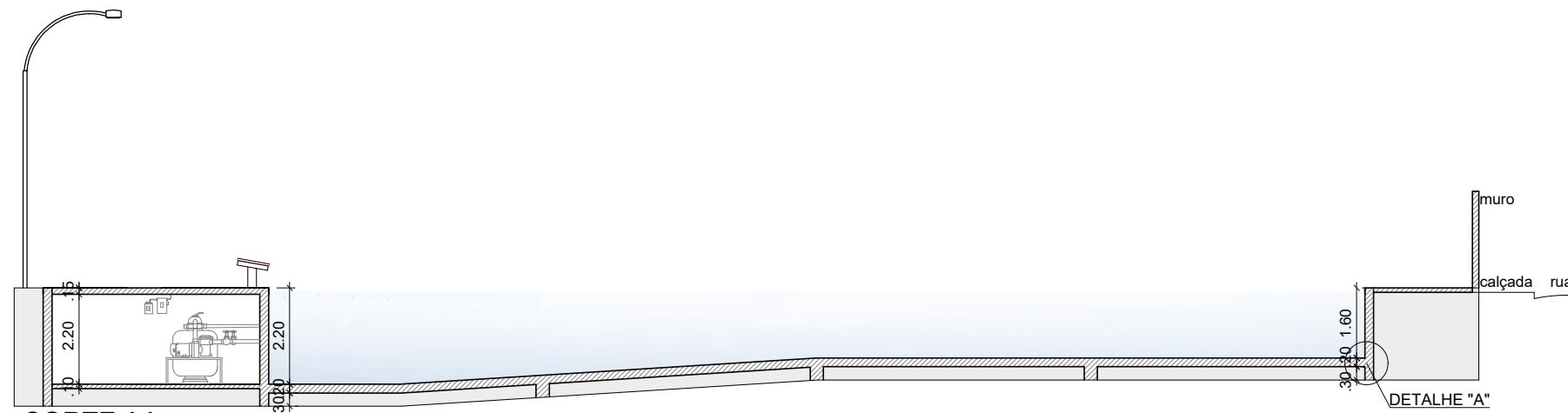
CORTE AA PISCINA SEMIOLÍMPICA escala 1/150 PREFEITURA DE JURUPIRANGA
