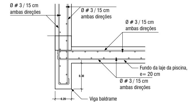
DETALHE "A"
