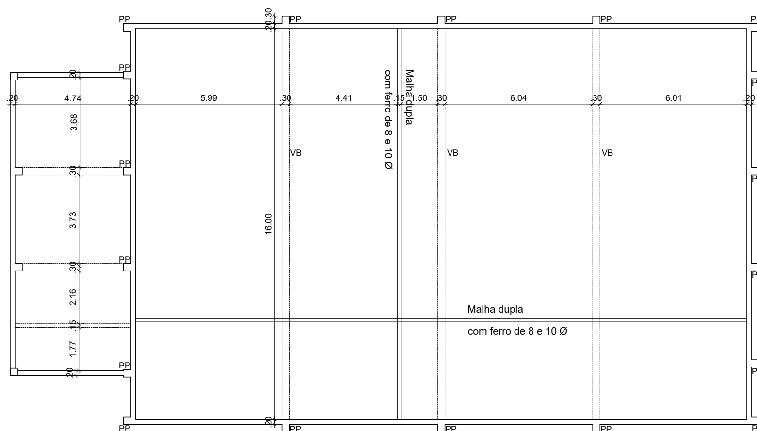
PLANTA ESTRUTURAL PISCINA SEMIOLÍMPICA PREFEITURA DE JURUPIRANGA escala 1/150
